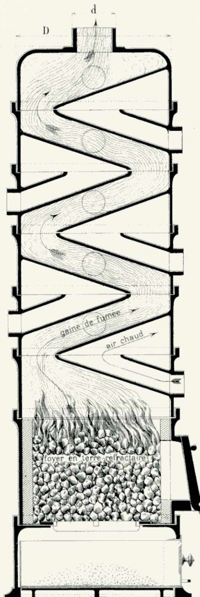
COUPE VERTICALE
